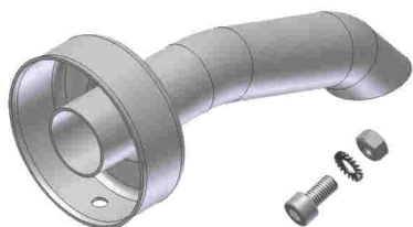
dB Killer Ø25 mm
